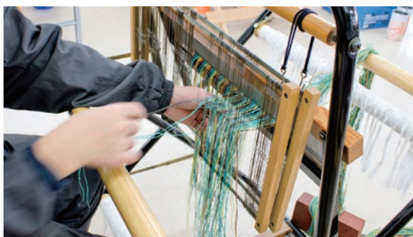
織り機に縦糸を通す作業は、さをり織りにおいて、一番神経を使います。
